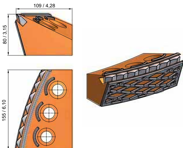
BRS13 BRS155x110x80 R
